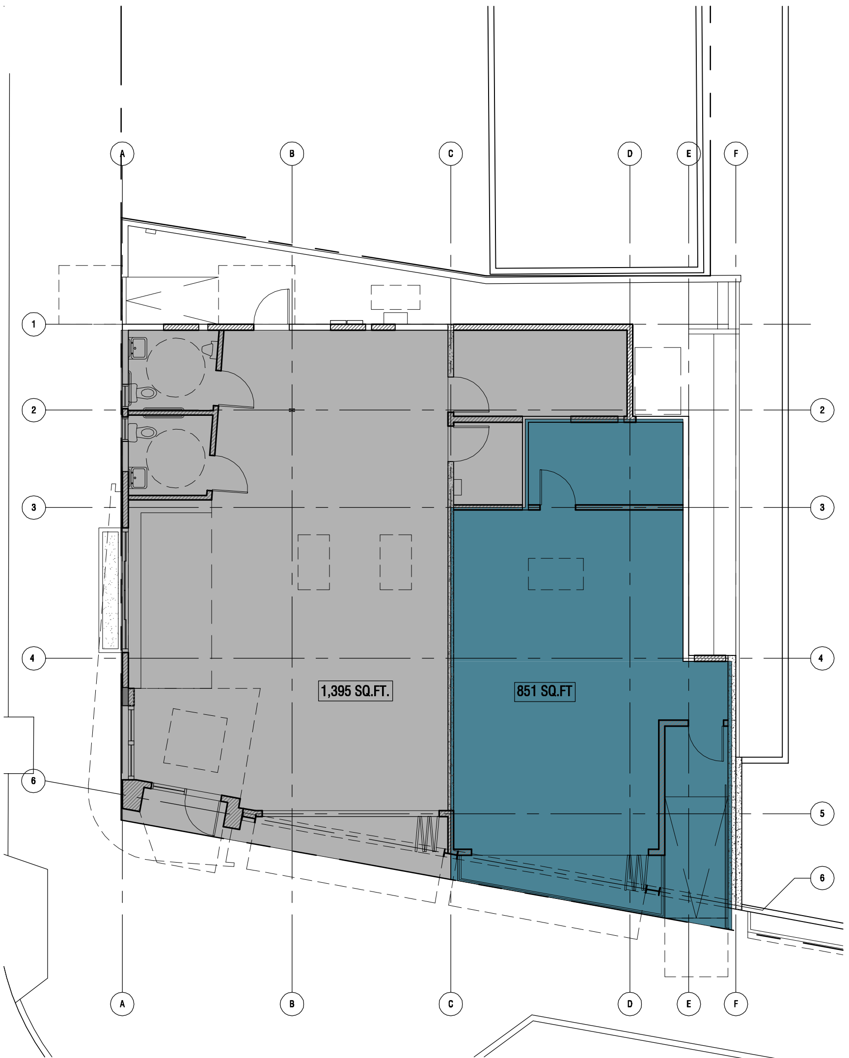
2 SOLANO FLOOR PLAN SCALE: 1/8" = 1'-0"
